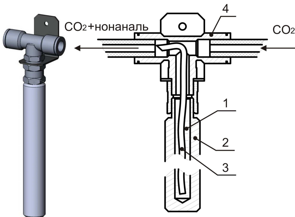
Рисунок 7 – модуль подмешивания аттрактанта в углекислый газ
